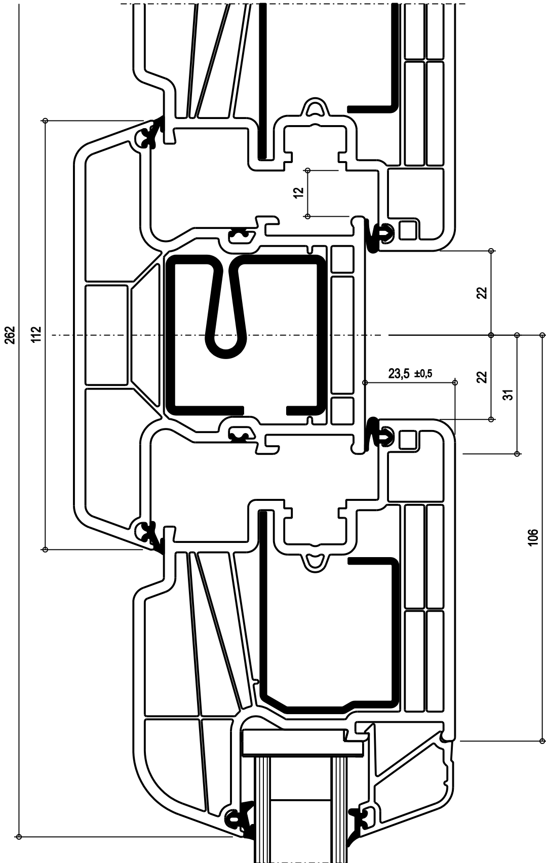
ZA 284/6D - 14526 Flügel vent frame vantail hoja battente
