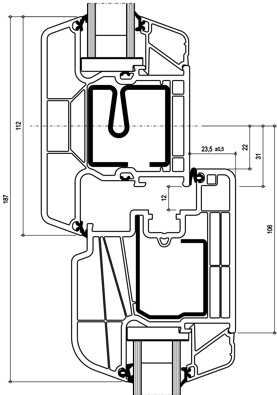
ZA 284/6D - 14526 Flügel vent frame vantail hoja battente
